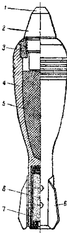
Рис. 3. Осколочная мина со взрывателем и вышибным патроном: 1-колпак взрывателя; 2-взрыватель; 3 - головная втулка; 4-корпус мины; 5-разрывной заряд; 6-крылья стабилизатора; 7-вышибной патрон; 8-пороховой заряд
